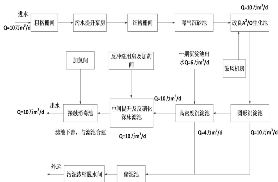
图 4-2 南区污水处理厂一、二期污水处理工艺流程图
