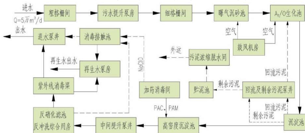
图 4-2 南区污水处理厂一、二期污水处理工艺流程图
