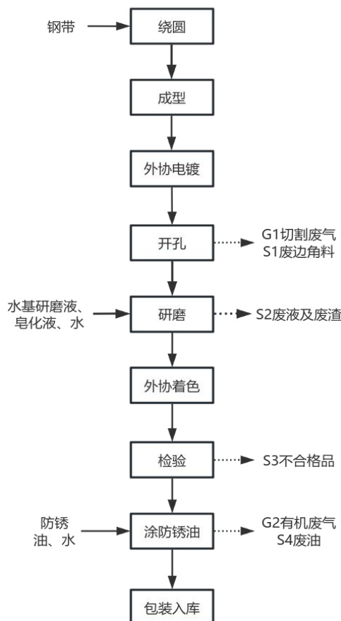
图 2-2 发动机活塞环生产工艺流程及产污节点图
