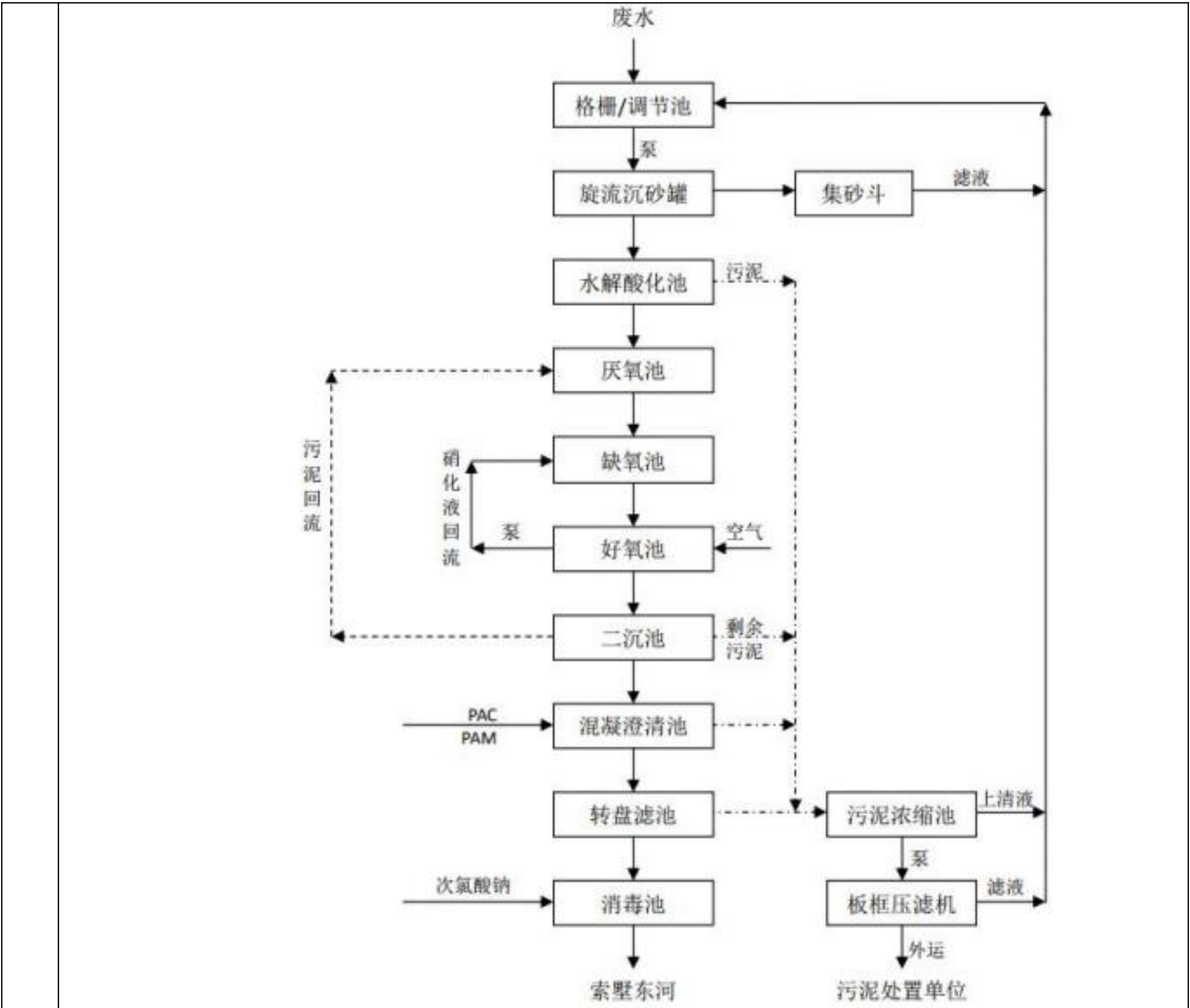
图 4-1 青龙污水处理厂工艺流程图
