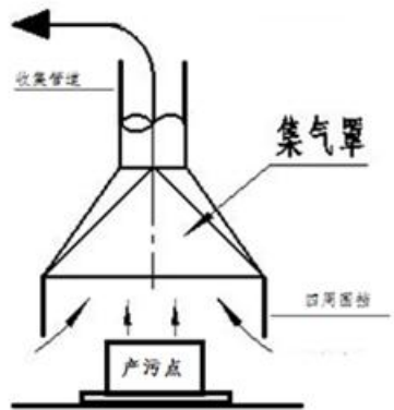
图 4-1 集气罩收集示意图
