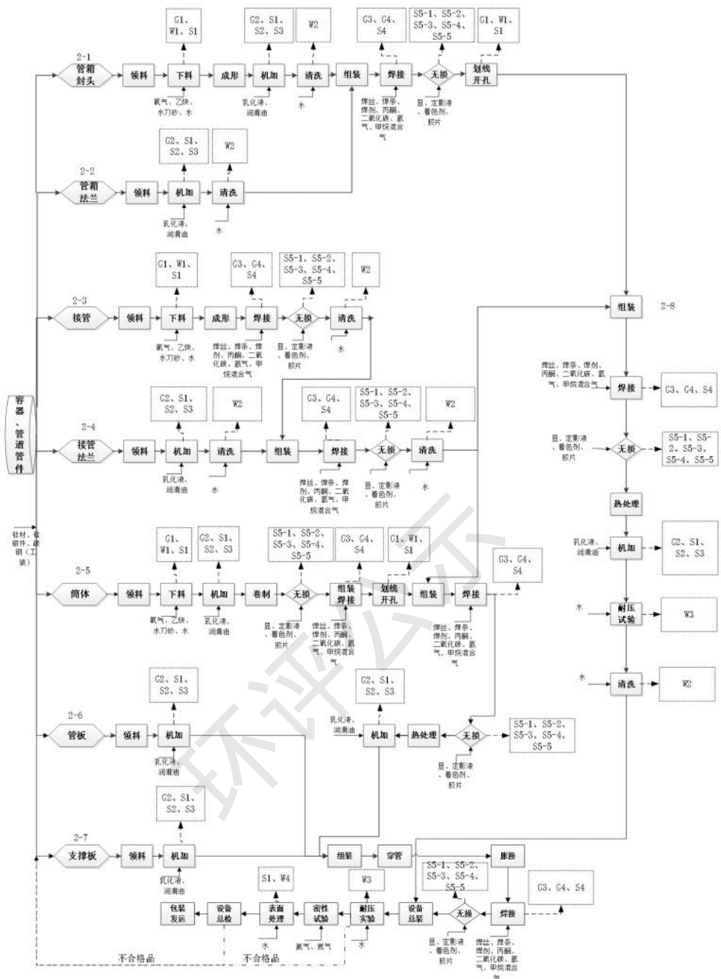
图 2-12 容器、管道管件工艺流程及产污节点图
