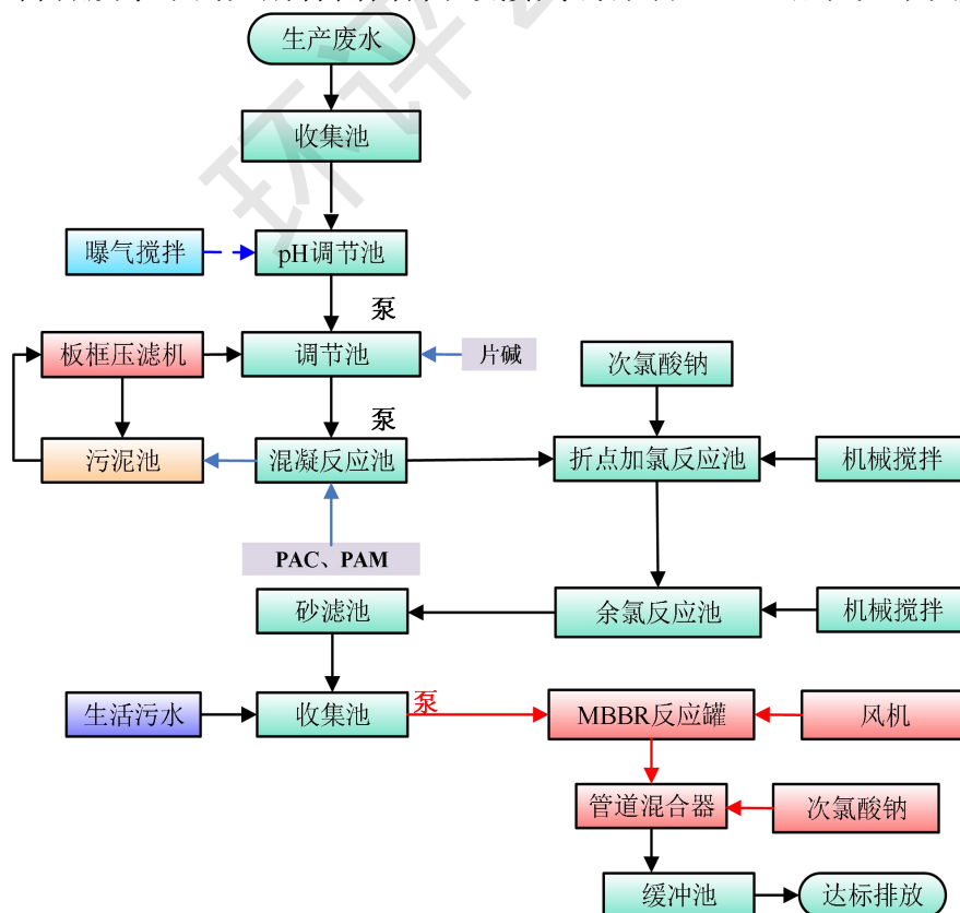
图 4-2 东厂区污水处理站工艺流程
