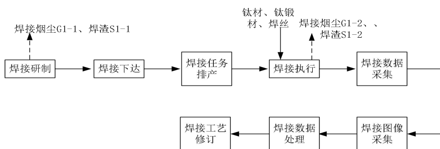
图 2-10 工业互联网+人工智能识别技术焊接工艺流程及产污节点图
