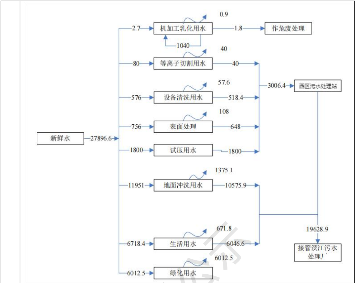
图 2-12 西厂区水平衡图 (t/a)
