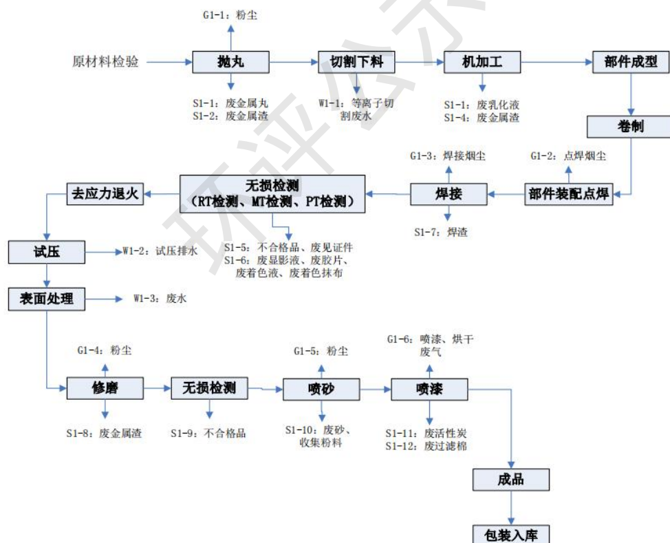
图 2-9 全厂超限装备（压力容器）生产工艺流程及产污节点图
