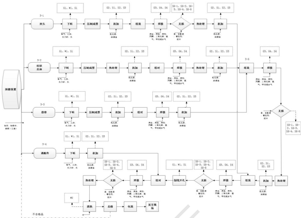
图 2-13 深潜装置工艺流程及产污节点图
