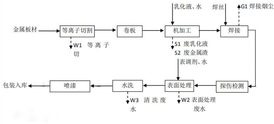
图 2-8 东厂区管道生产工艺流程及产污节点图
