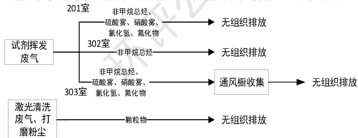
图 4-1 本项目废气收集处理流程图
