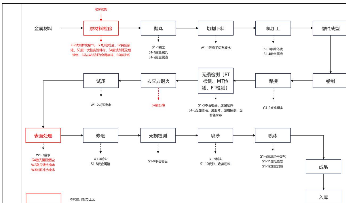
图 2-3 东厂区压力容器生产工艺流程及产污节点图
