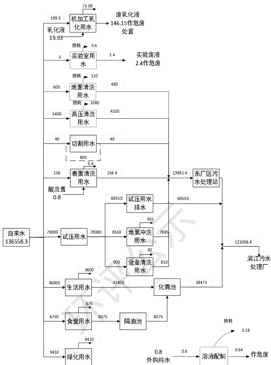
图 2-1 本项目实施后东厂区水平衡图 (t/a)
