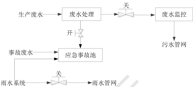
图 4-6 事故废水/消防尾水防范和处理流程示意图
