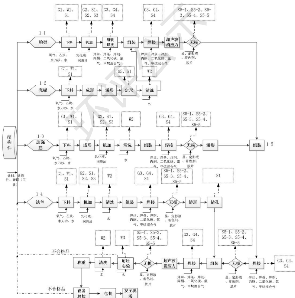
图 2-11 结构件（胎架、壳板、加强筋、法兰）工艺流程及产污节点图
